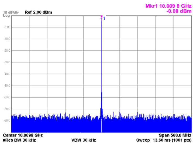
杂散测试
